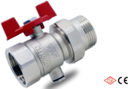
Klorimetre Isı Vanası - Dış Dişli, Kelebek Kollu, PN10
