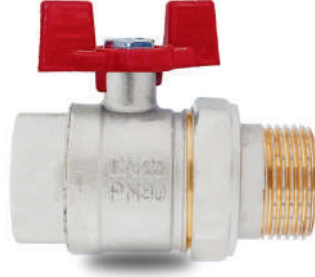
Kollektör İçin, Dış Dişli, Küresel Vana PN25 (Ağır Tip)
